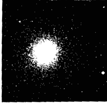
(དཔེ་རིས་ ༤ ང་ཚོའི་སྐར་ཚོགས་ཀྱི་དབུས་ཀྱི་ཉི་འགམ་དུ་ཡོད་པའི་རྒྱ་སྐར་ཀྱི་ཚོམ་བུ་ཞིག དེ་ཚོའི་རྒྱུང་ཚད་ནི་ས་གཞི་ནས་འོད་ལོ་སུམ་ཁྲི་འཕམ་མི་ཉེས་ ༧ x 10 10 ཙམ་ཡོད།)
