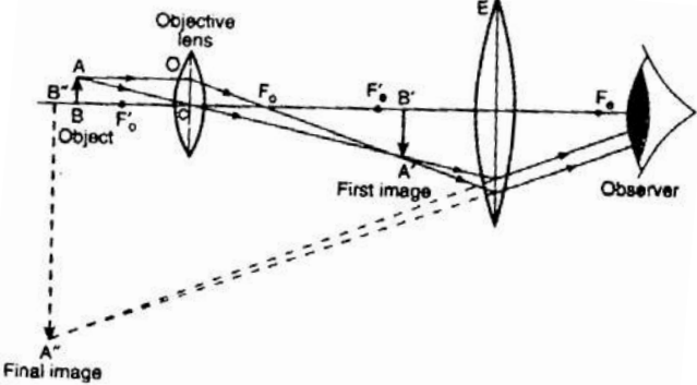
(དཔེ་རིས་ ༡༥ : སྤྱི་མཐོང་ཆེ་ཤེལ་ཞིག་གི་འདྲ་གནས་རིང་ཚད།)
