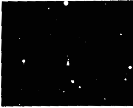
(དཔེ་རིས་ ༤ ལྷོ་ལོ་ ༡༩༧༠ རང་རྒྱུ་ཤེལ་ཡིན་ཆེ་ཉེས་བརྒྱ་ཡོད་པ་གཅིག་གི་བརྒྱུད་ནས་རྒྱུ་ཐག་རིང་ ཤོས་ཀྱི་དངོས་པོ་དེ་བྱུ་ཏེས་(Bootes)རང་ ༣༨༧༧ (མདས་མཚོན་པར་བྱས་) ནས་ཚད་འཇལ་བྱས་ཡོད།)
