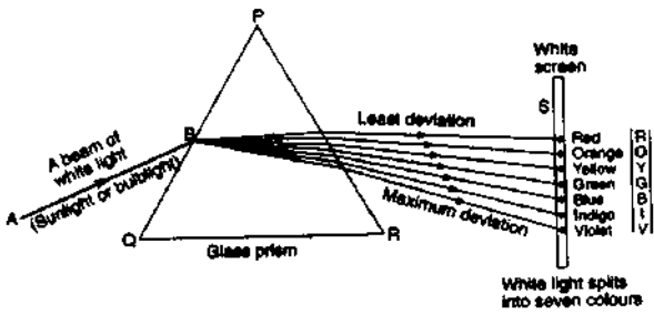
(དཔེ་རིས་ ༧།: འཇའ་ཤེལ་ཞིག་གིས་འོད་དཀར་པོ་ཞིག་ཁ་དོག་བདུན་དུ་གྲམ་པ་ཡིན།)
