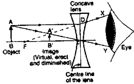
(དཔེ་རིས་ ༡། : ཀོང་ཤེལ་ཞིག་གིས་གཟུགས་བརྟན་གྲུབ་ཚུལ།)
