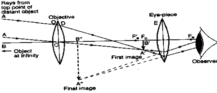
(དཔེ་རིམ་ ༣༧ : སྐར་དབུད་རྒྱང་ཤེལ་ཞིག་གི་འོད་འཕྲོའི་རིམ་ལོ།)
