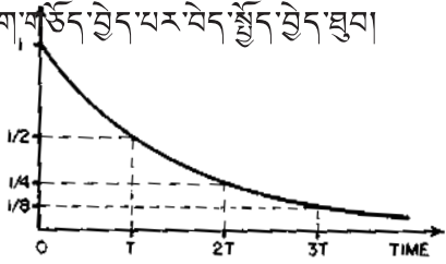
(དཔེ་རིས་ ༡ རེ་རྩེའོ་ ཨེག་ཤི་ཕི་ཤི་དང་དུས་ཀྱི་ཐིག་རིས།(The decrease with time of radioactivity)ཚེ་སྲིད་(half-life)རེ་རེའི་ནང་སྲིད་གཅིག་(one-half)ཚོད་ཀྱིས་ཉམས་ཏེ་འགོ་བ།(The activity decreases by one half in each "half-life", T.)
