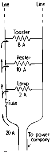
(དཔེ་རིས་ 11 ཁང་པའི་ རང་སློབ་མཁོ་སྤོང་བྱེད་མཁུ་ ལུ་དབྱིན་ལ་མཐུད་པའི་ཡོ་ ཆས་ཀྱི་རྒྱ་ལམ་གྱི་རི་མོ།)
